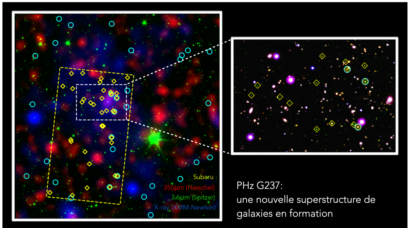
Région du ciel montrant le proto-amas de galaxies G237 lorsque l'univers était âgé d'environ 3 milliards d'années. © ESA/Herschel and XMM-Newton; NASA/Spitzer; NAOJ/Subaru; Large Binocular Telescope; ESO/VISTA; Polletta et al. 2021; Koyama et al. 2021.
